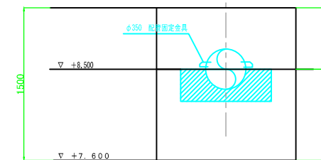
C-C断面 (S=1/20)
