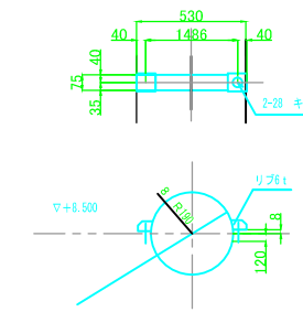
φ350 配管固定金具詳細図(4ヶ所) S=1/10
