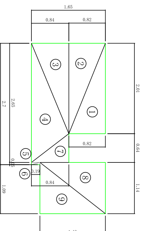
調理場求積図 S=1/500
