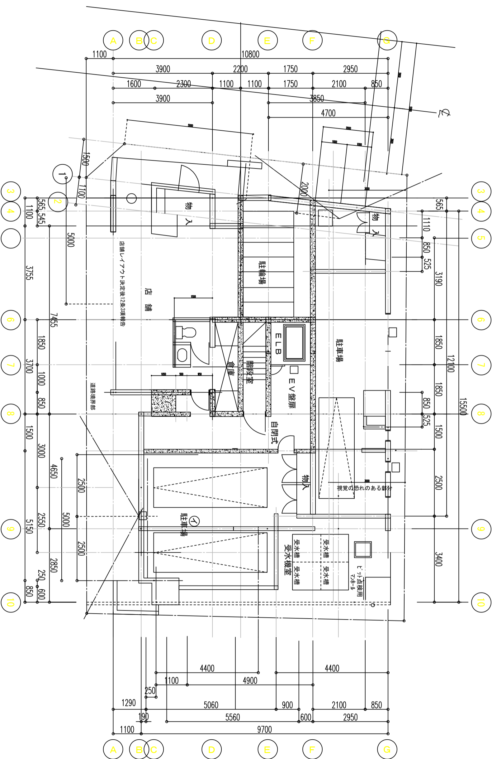
1階平面図 S=1:100
