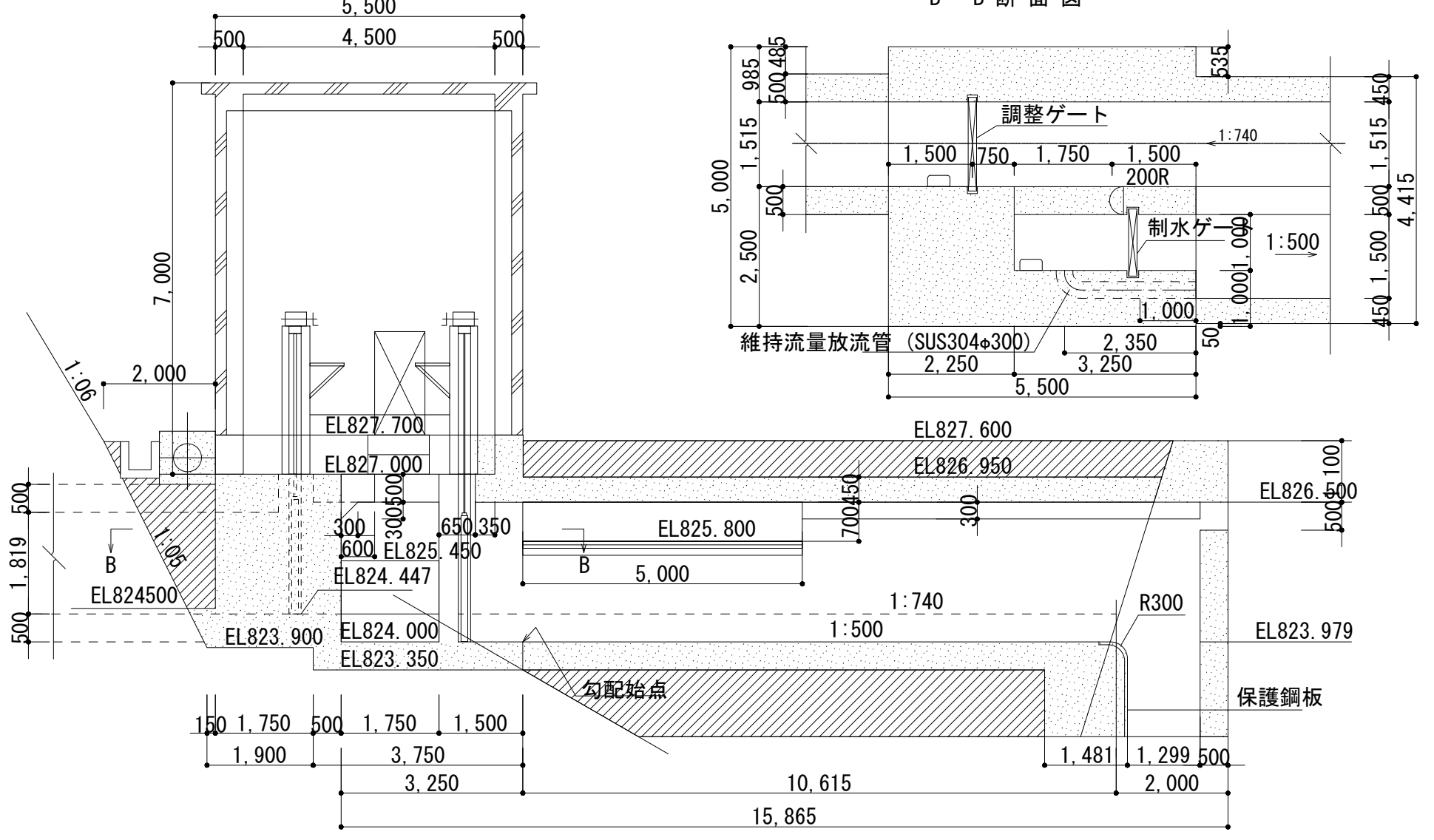
A-A断面図
