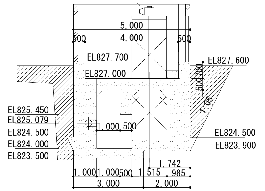
D-D断面図
