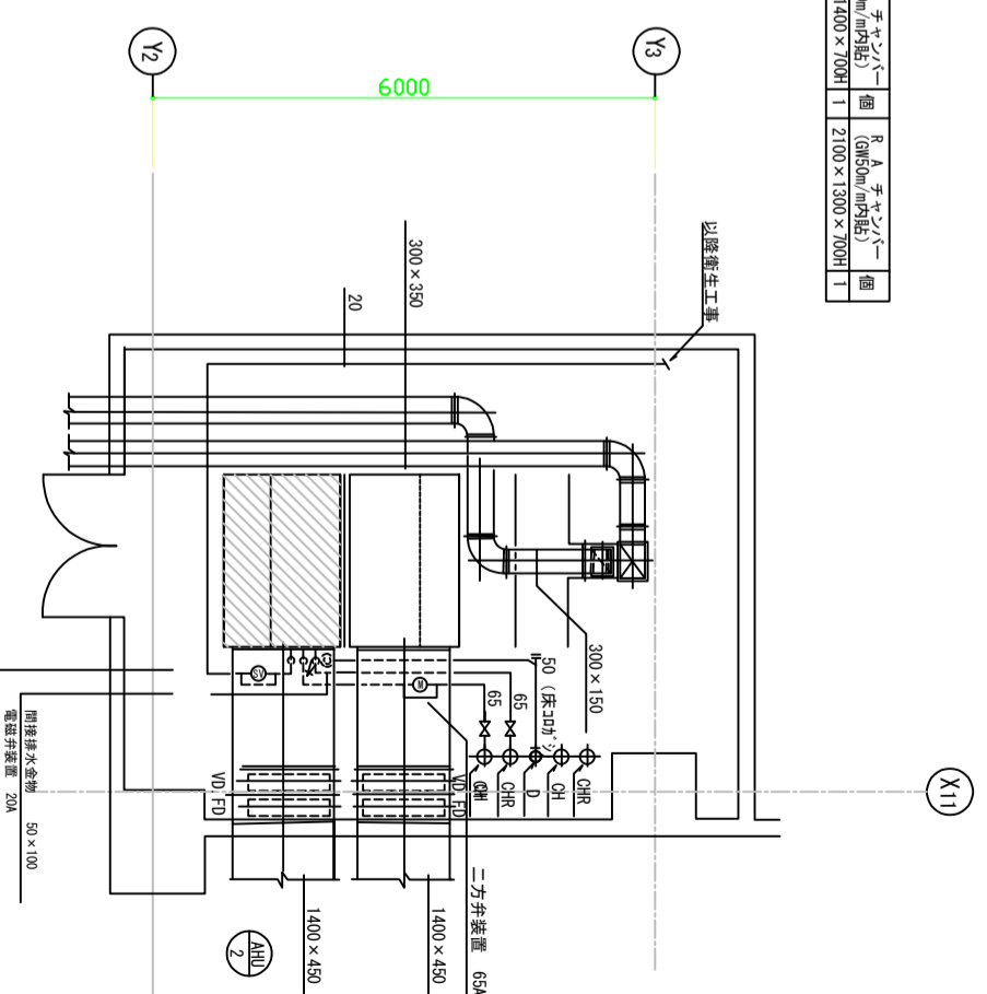
B1F 空調機機室 (3) 平面詳細図 S=1:50
