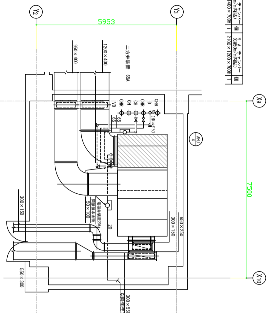
B1F 空調機機室 (4) 平面詳細図 S=1:50
