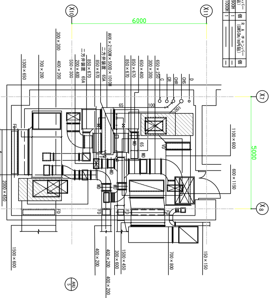
B1F 空調機機室 (1) 平面詳細図 S=1:50
