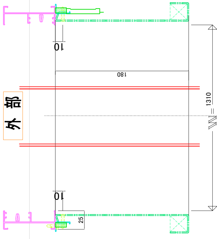
平面図
