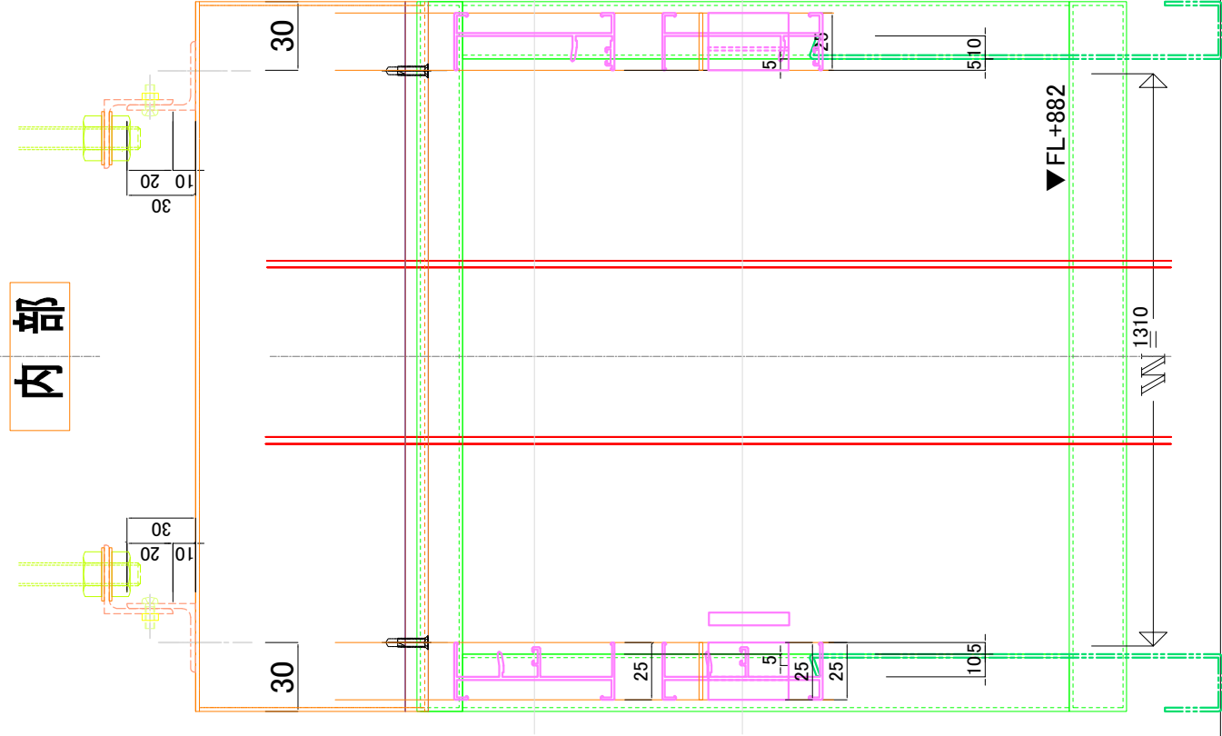
正面図
