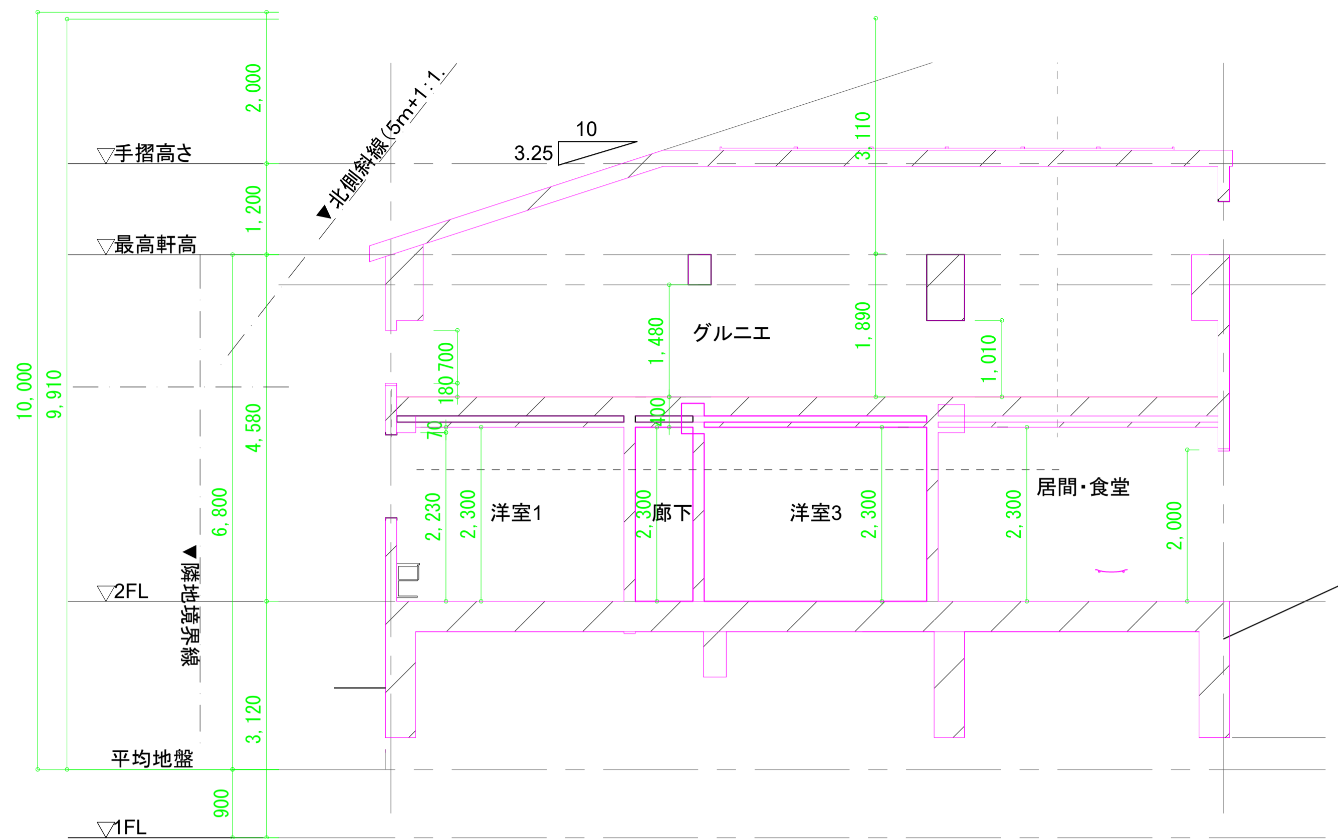
Y1-Y1'断面図 S=1:100
