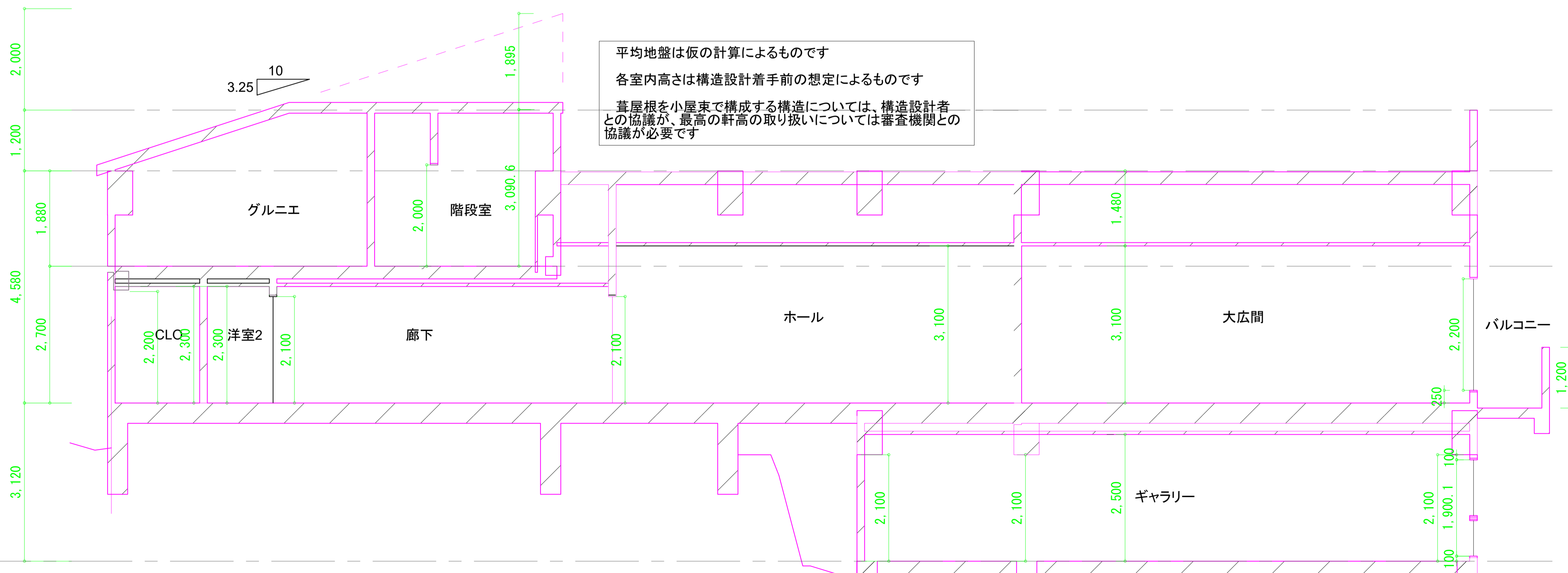
X-X'断面図 S=1:100
