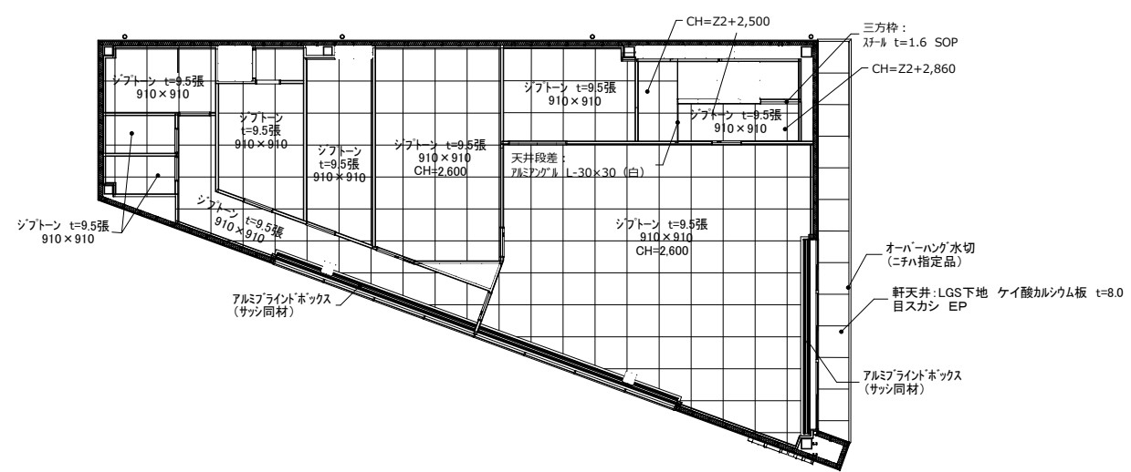
2階天井伏図 S=1:100
