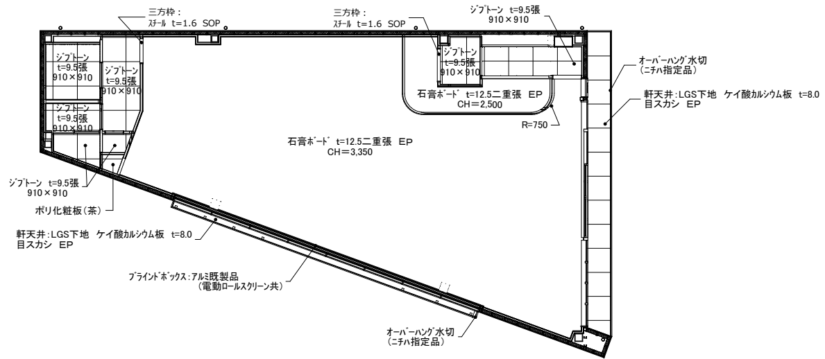
1階天井伏図 S=1:100
